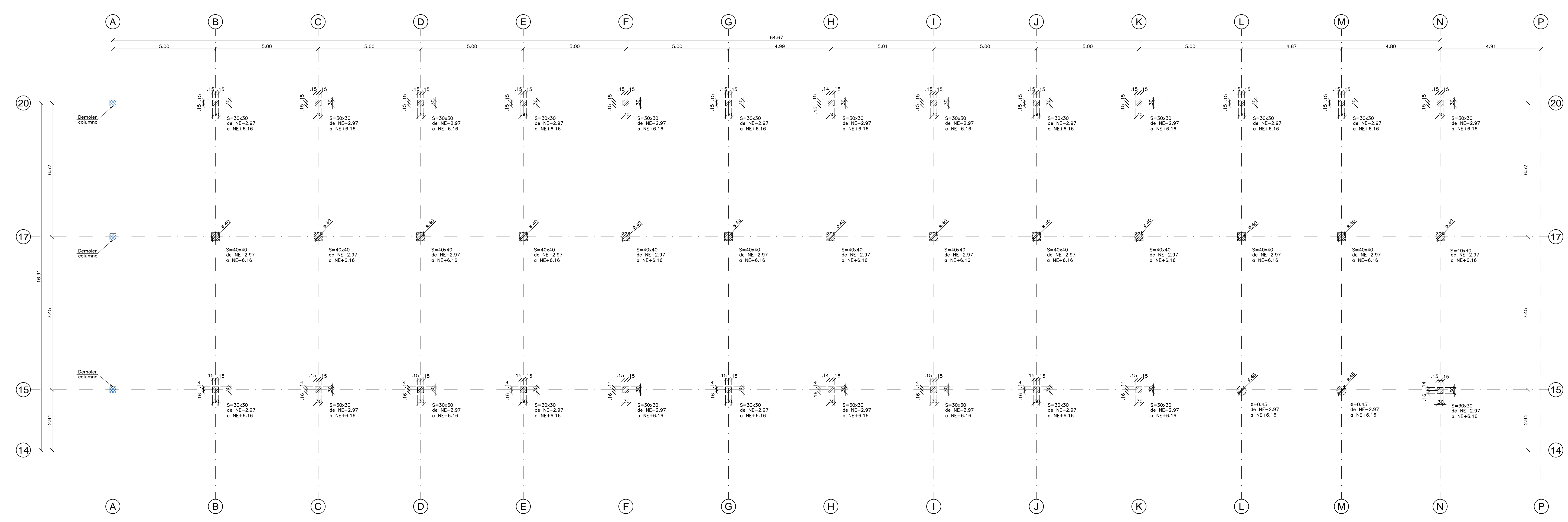
ESTRUCTURA 2 BLOQUE 2 - PLANTA LOCALIZACIÓN DE COLUMNAS - DEMOLICIÓN ESCALA 1:100
